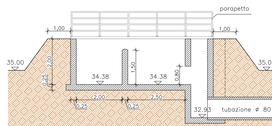
SEZIONE A-A (1:100)
