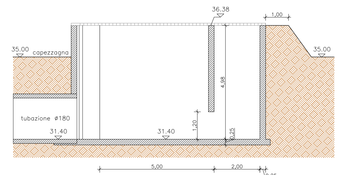
SEZIONE C-C (1:100)
