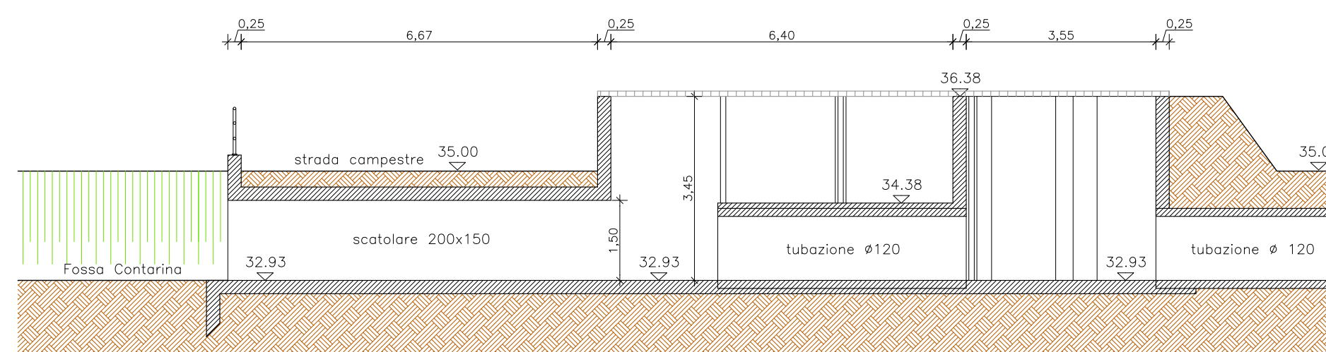
SEZIONE B-B (1:100)
